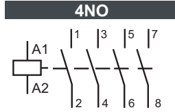
Bağlantı Şeması:
