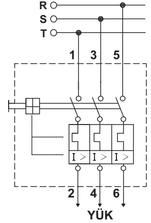
Bağlantı Şeması
