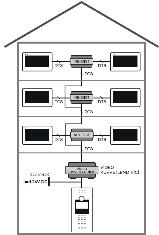
MULTIBUS BUAT TİPİ UYGULAMADA KABLOLAMA
